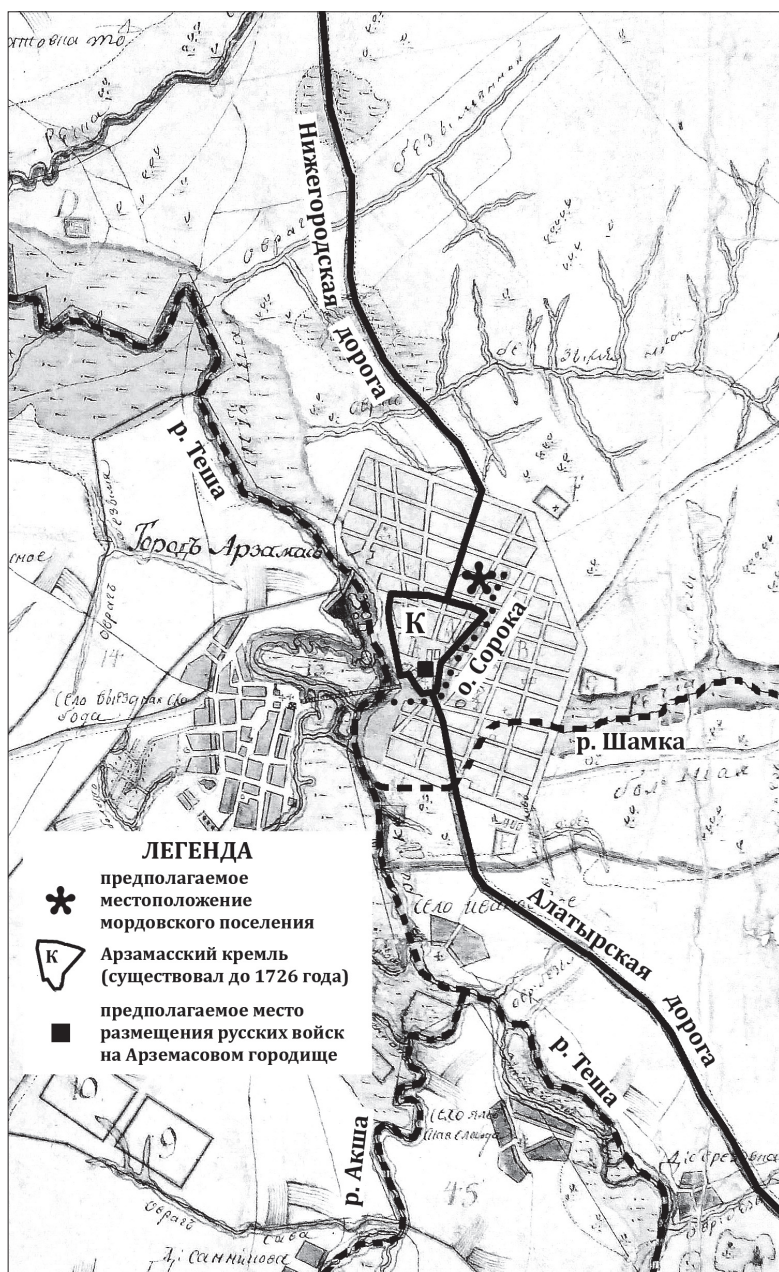
Иллюстрация III. Арзамас на плане генерального межевания 1791 года
